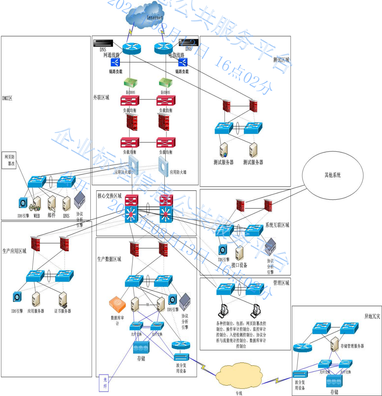
图 B.1 增强网络安全防护架构参考图
